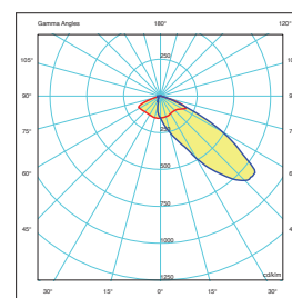
Asimmetrica Concentrante
