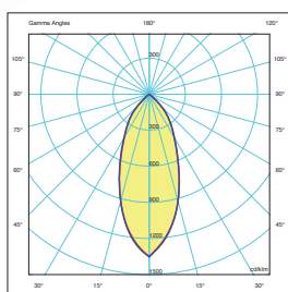
Rotosimmetrica concentrante
