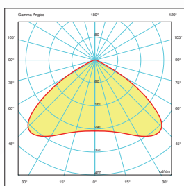
Rotosimmetrica diffondente
